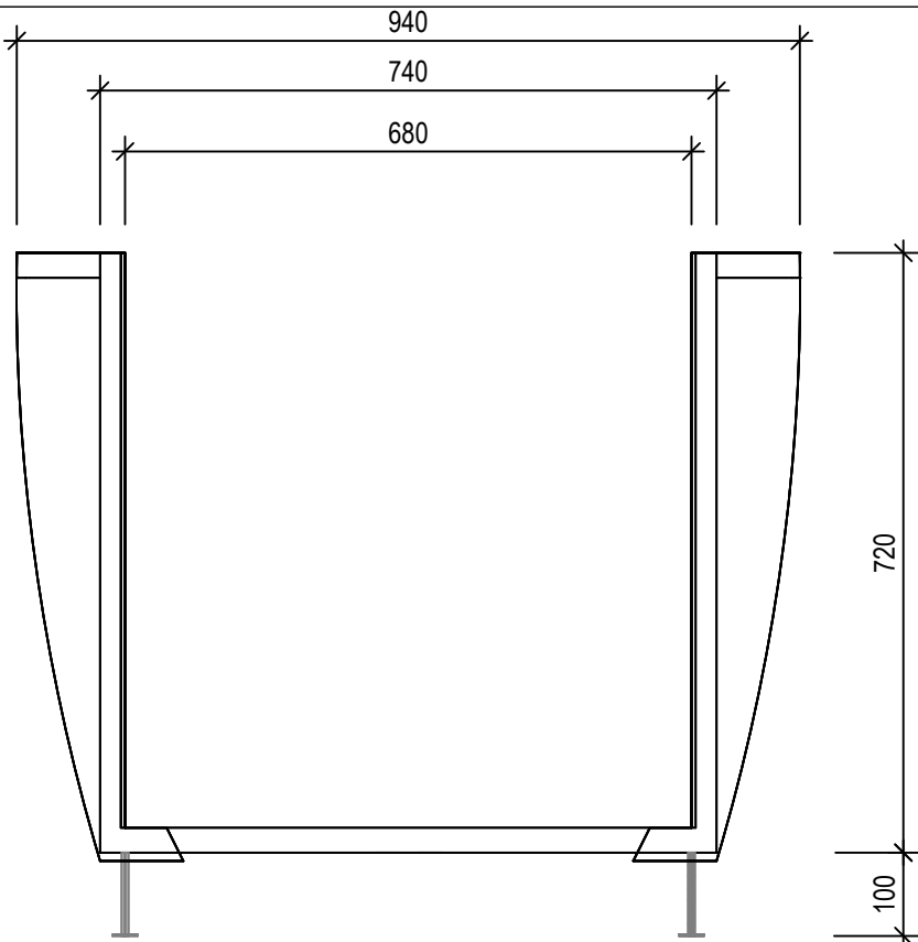
Frontansicht
